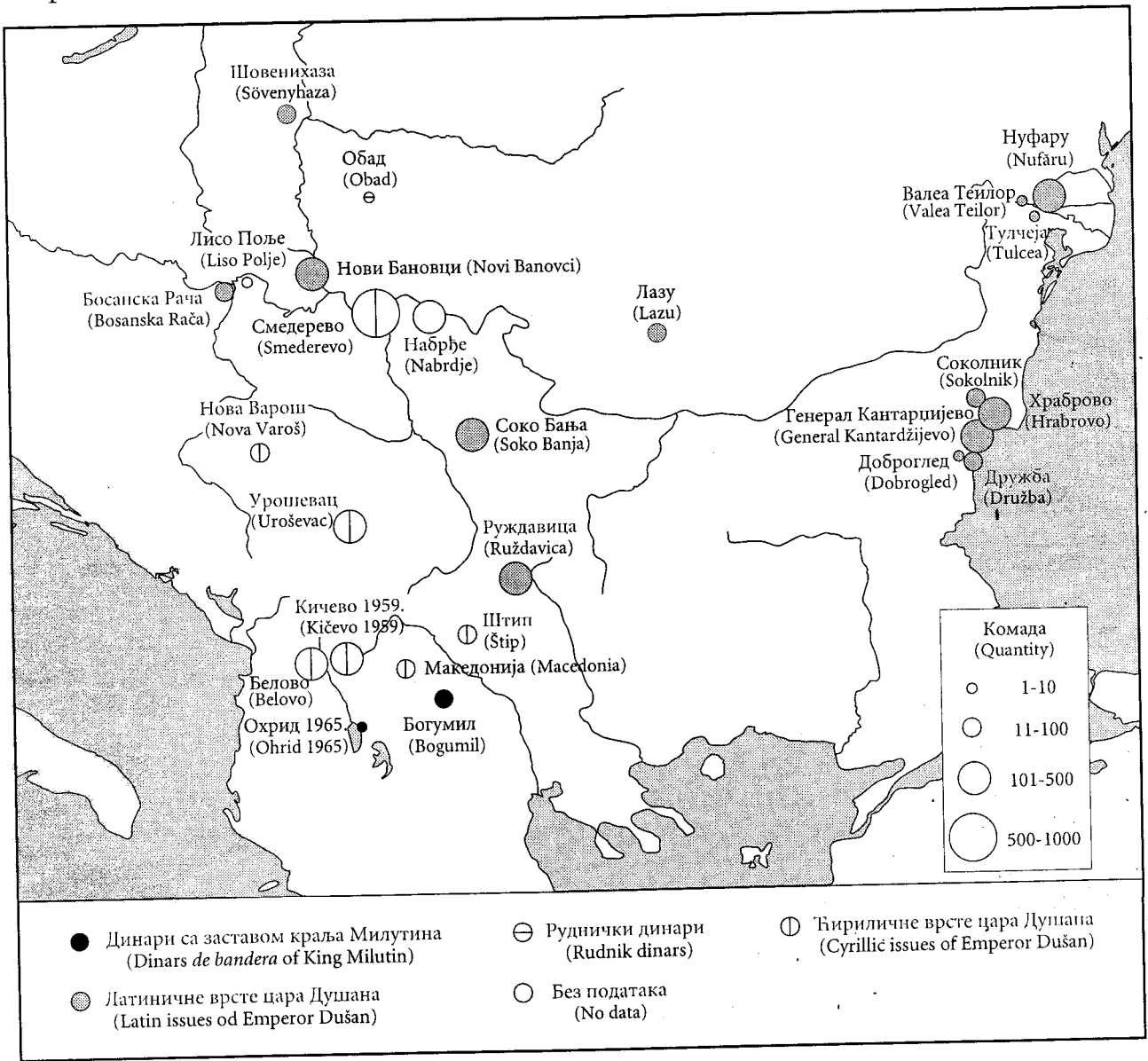
Карта 5: Остатке са српским динарима похрањене између 1346. и 1355. године Map 5: Hoards with Serbian dinars deposited between 1346 and 1355
