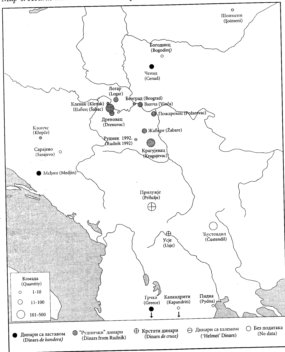
Карта 4: Остаци са српским динарима похрањене између 1315. и 1346. године Map 4: Hoards with Serbian dinars deposited between 1315 and 1345
