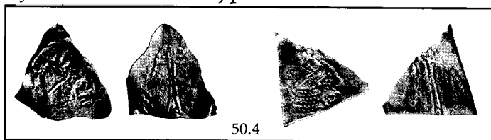
Слика 3: Неопредељени динари из времена Вука Бранковића - врста 50.4 Illustration 3: Uncertain dinars from the time of Vuk Branković - type 50.4
