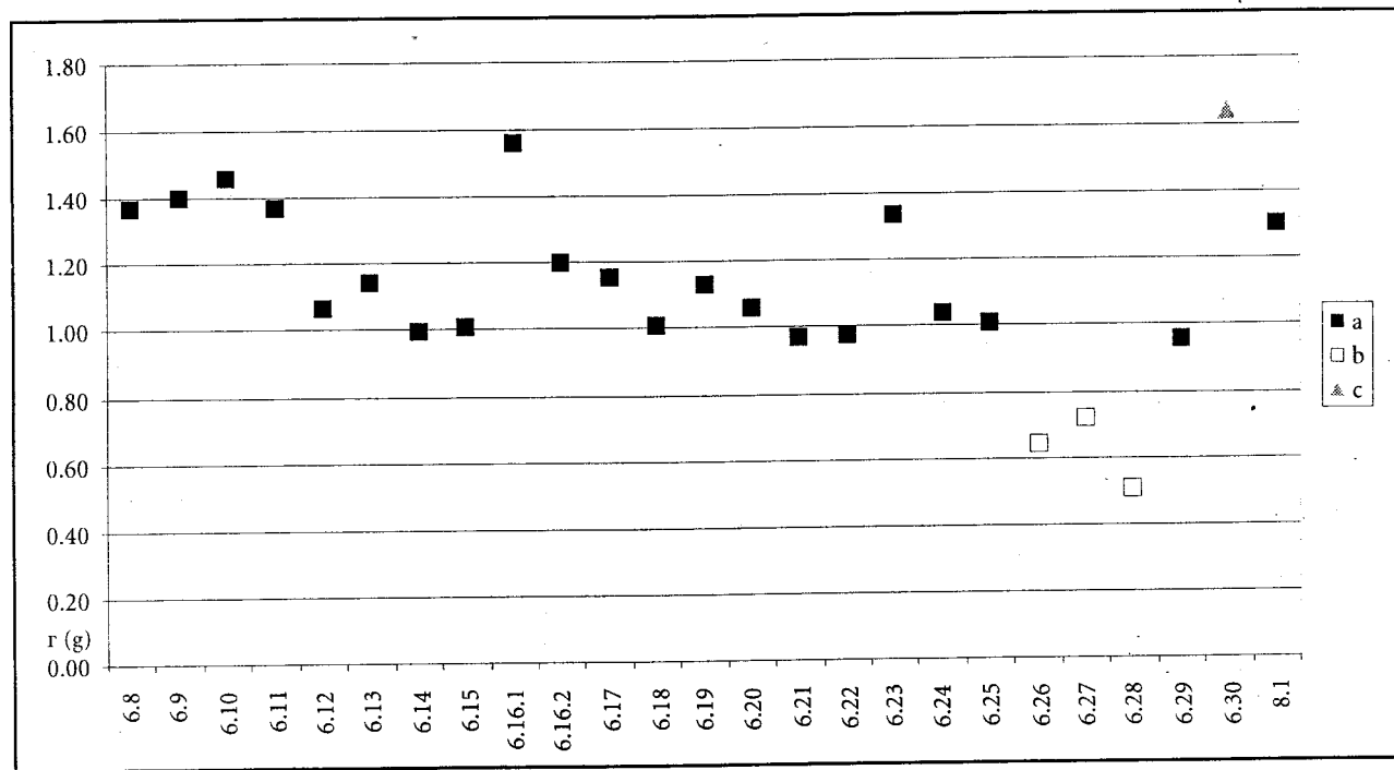
Графикон 5: Средње тежине новца из времена цара Уроша:
