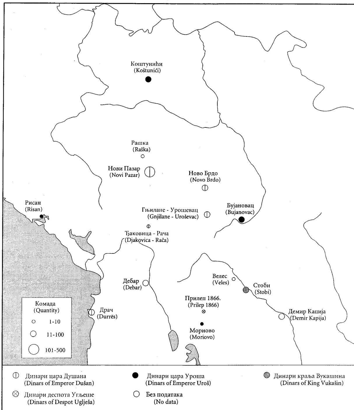
Карта 6: Остатке са српским динарима похрањене између 1355. и 1371. године Map 6: Hoards with Serbian dinars deposited between 1355 and 1371
