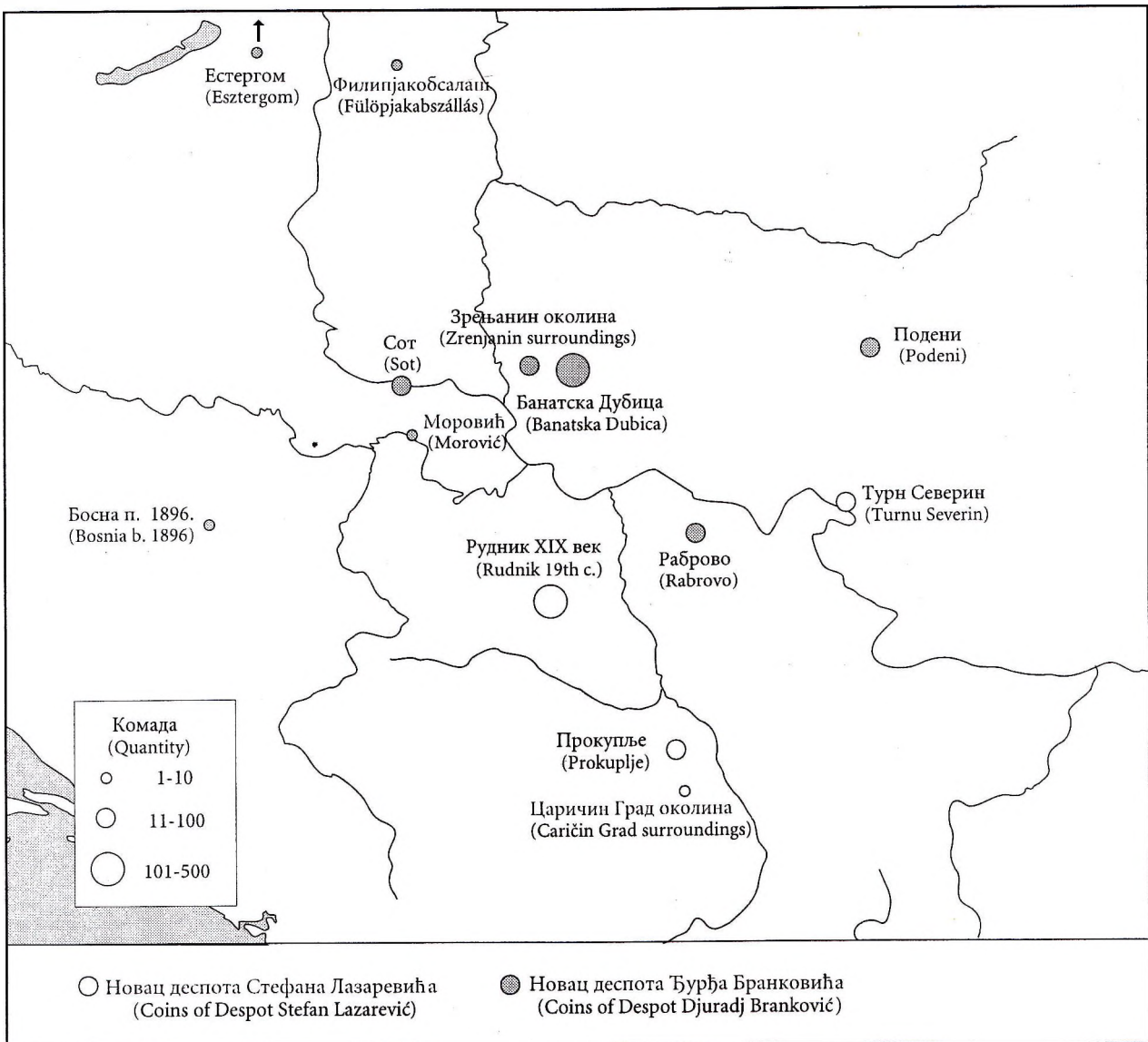
Карта 9: Оставе са српским динарима похрањене између 1402. и 1456. године Map 9: Hoards with Serbian dinars deposited between 1402 and 1456
