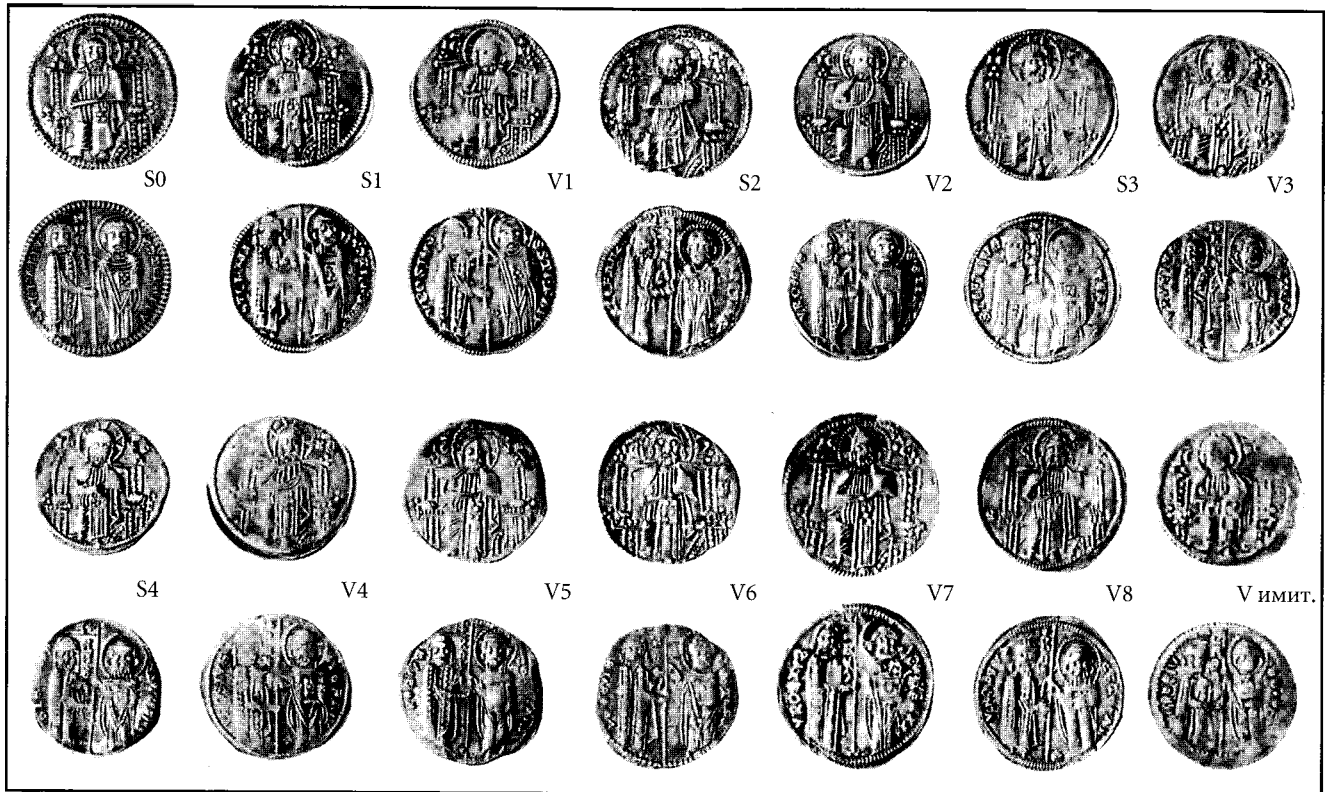
Слика 5: Емисије динара са заставом краљева Драгутина и Милутина Illustration 5: Issues of dinars 'de bandera' of kings Dragutin and Milutin
