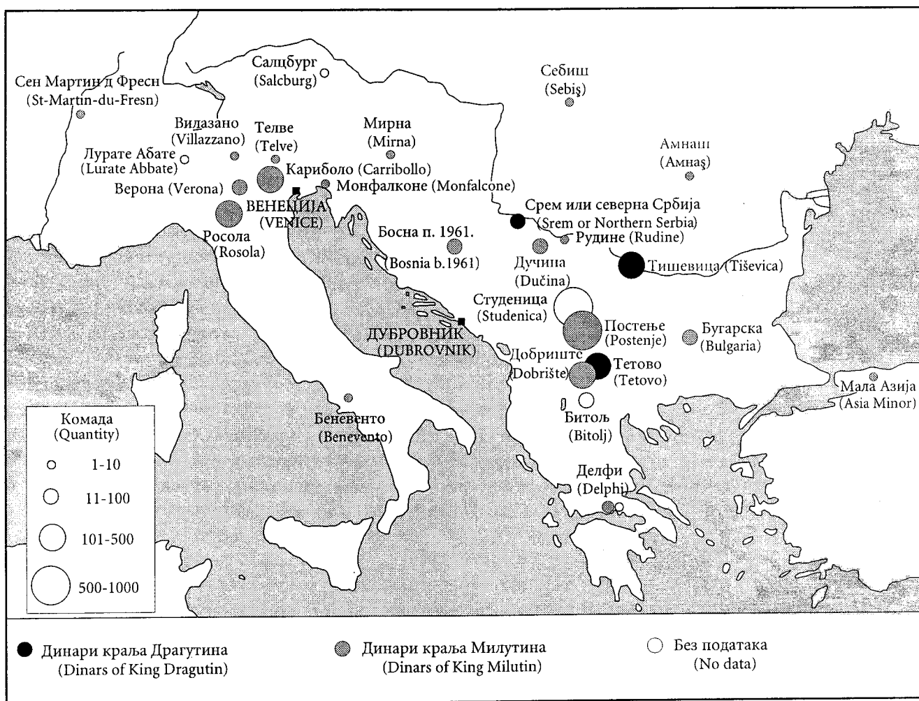
Карта 3: Осипаве са српским динарима са зашћавом похрањене између 1280. и 1325. године Map 3: Hoards with Serbian dinars 'de bandera' deposited between 1280 and 1325
