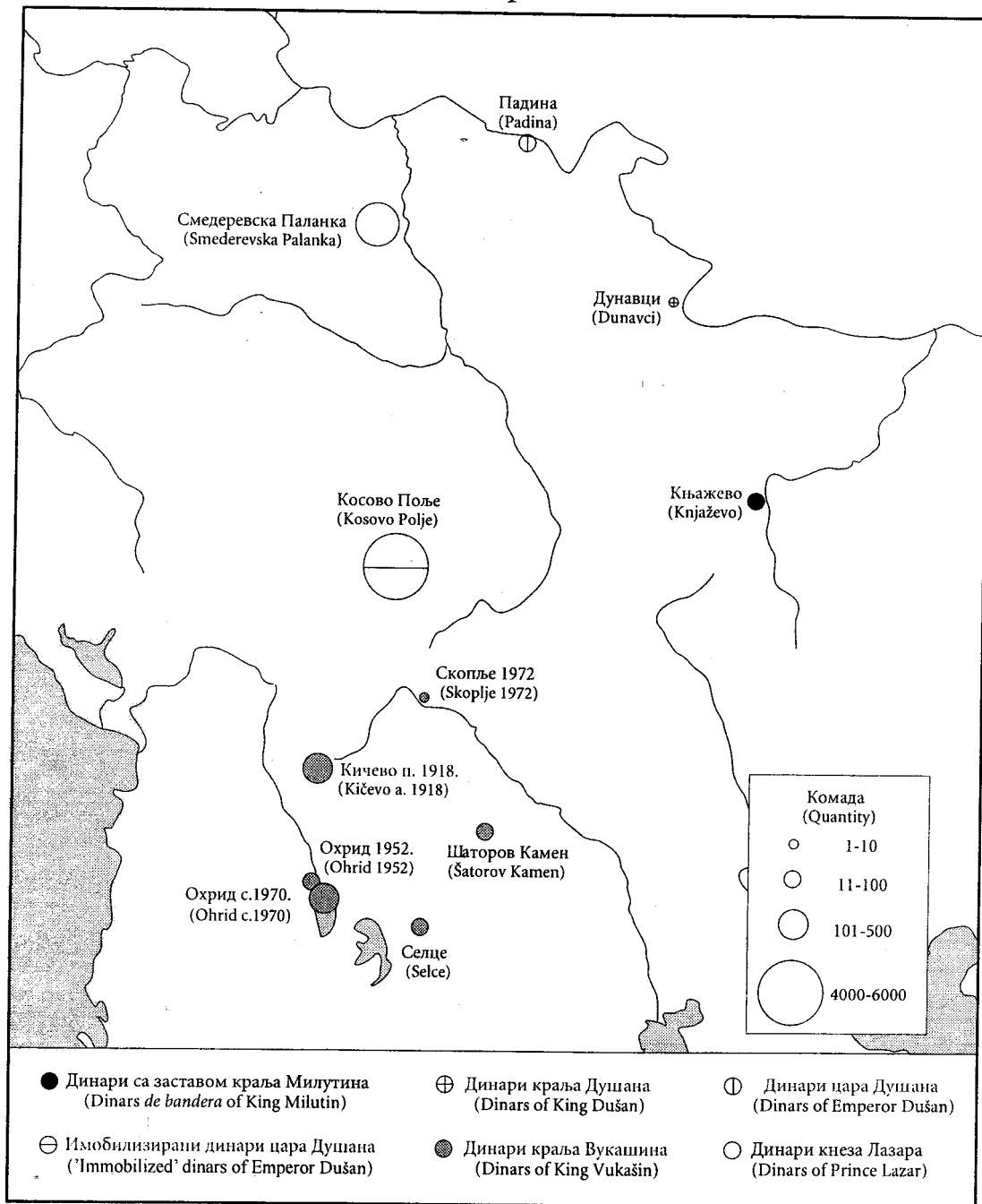
Карта 7: Остаци са српским динарима похрањене између 1371. и 1380. године Map 7: Hoards with Serbian dinars deposited between 1371 and 1380
