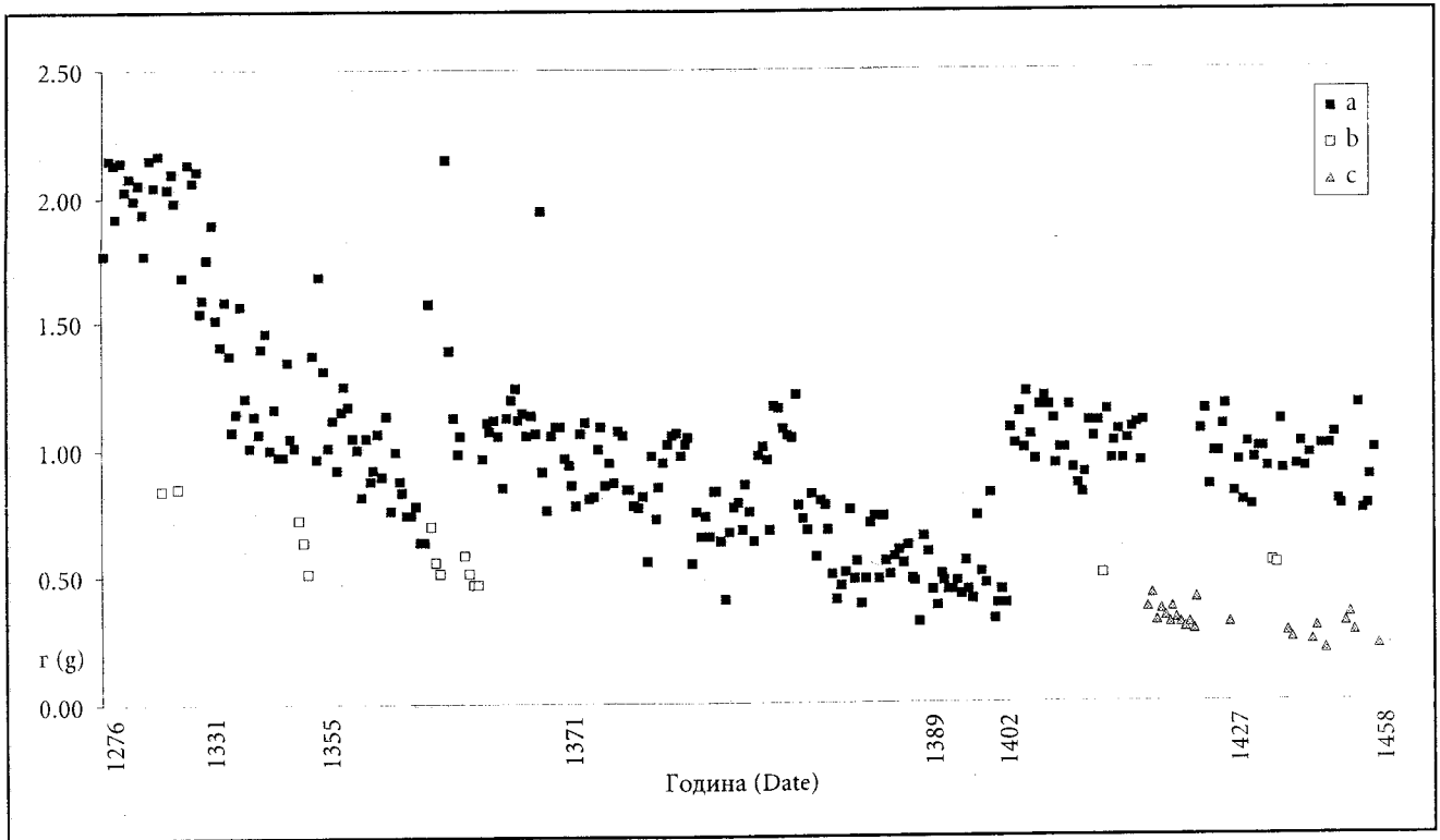
Графикон 1: Средње тежине српског новца: а) Динари; б) Полудинари; с) Оболи Chart 1: Average weights of Serbian coins: а) Dinars; б) Half-dinars; с) Oboli
