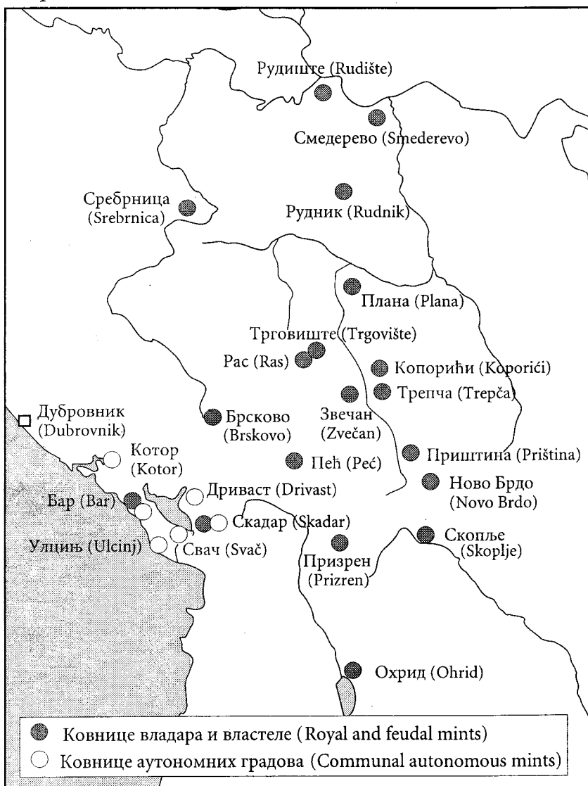
Карта 2: Ковнице новца у средњовековној Србији Map 2: Mints in medieval Serbia
