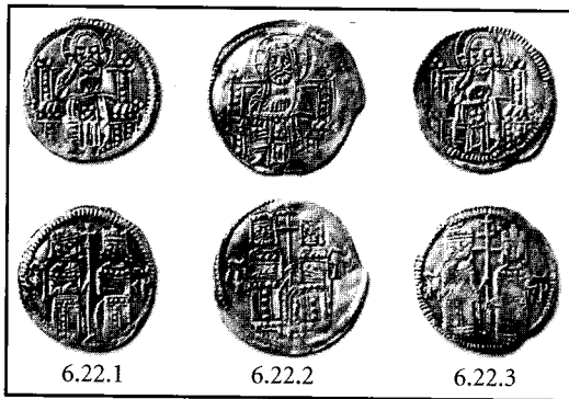
Слика 12: Ковања врсте 6.22 на различитим плочицама Illustration 12: Coinages of the type 6.22 on different flans
