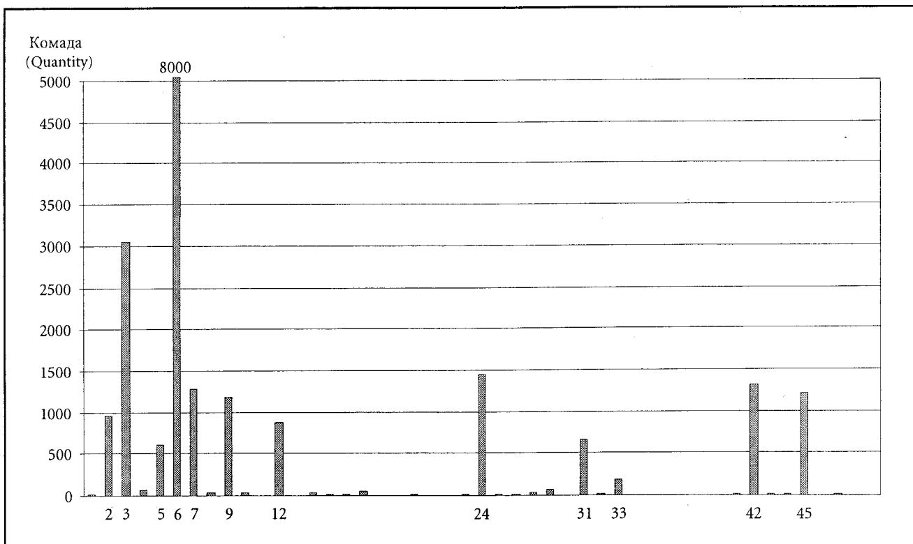
Графикон 2: Број сачуваних примерака новца у оставама, збиркама и појединачним налазима Chart 2: Number of surviving coins in hoards, collections and single finds
