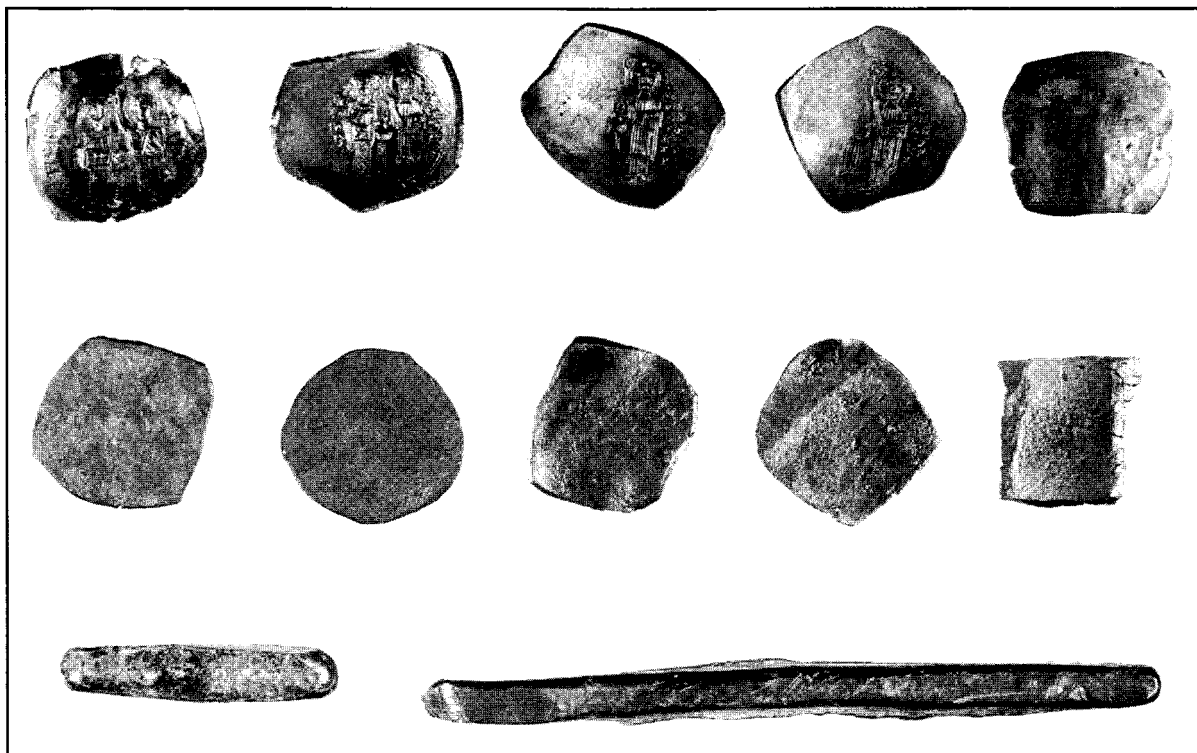
Слика 1: Билон трахеји, њлочице и слийиак за ковање новца краља Сийефана Рагослава Illustration 1: Billon trachea, flans and ingots for minting coins of King Radoslav
